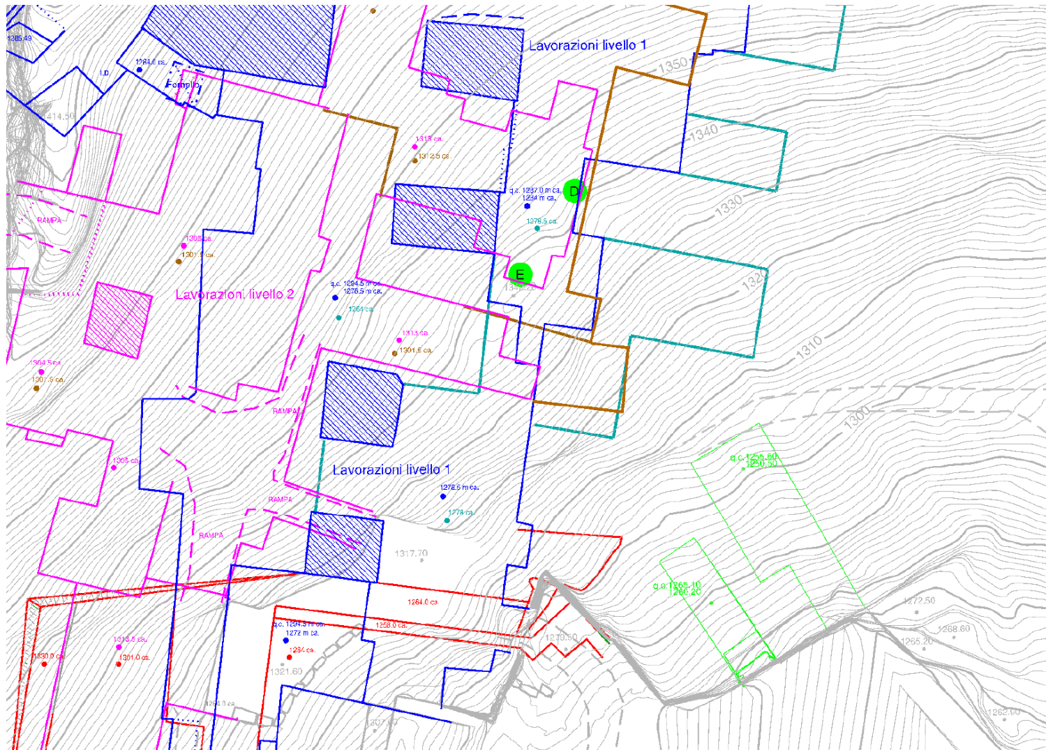
Estratto tavola perizia giugno 2021 con indicate le fratture beanti D ed E a livello 2
